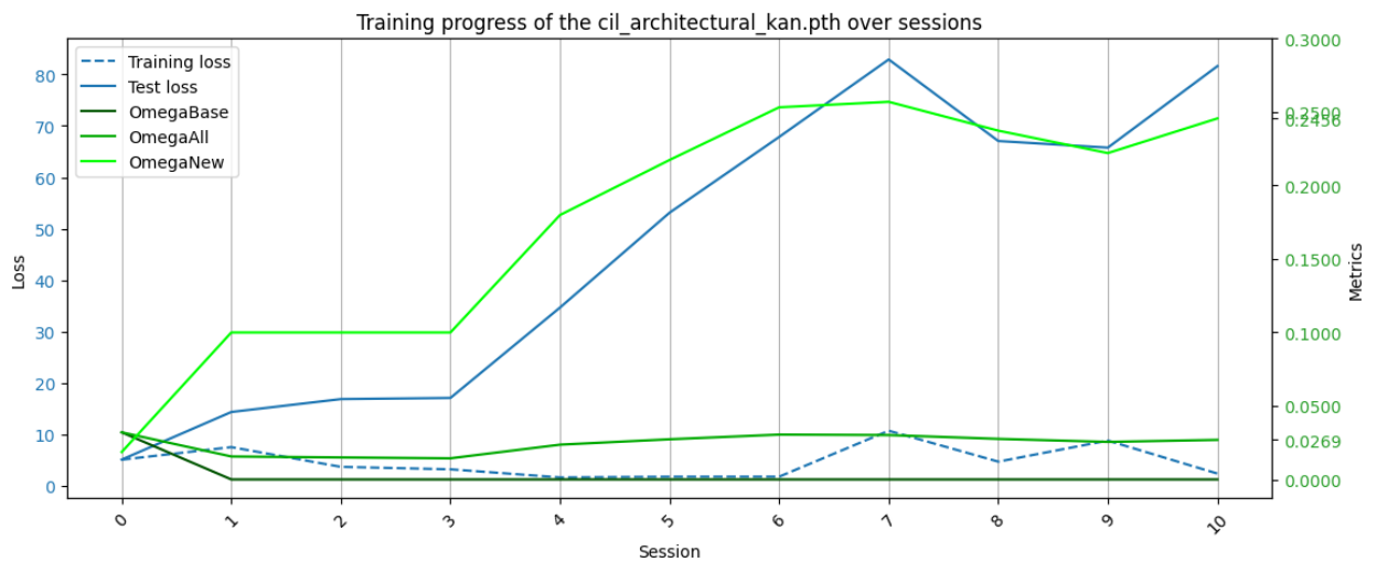
Приложение 12: График обучения KAN с адаптированным FEL в эксперименте с инкрементальным обучением классам
