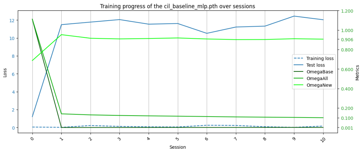
Приложение 10: График обучения MLP в эксперименте с инкрементальным обучением классам
