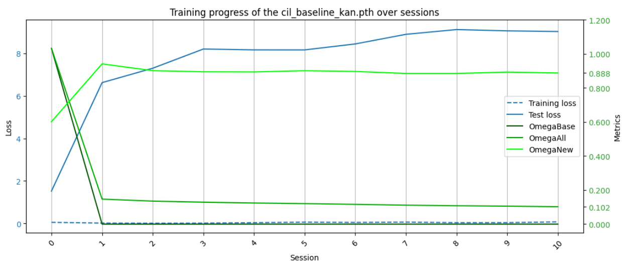
Приложение 11: График обучения KAN в эксперименте с инкрементальным обучением классам
