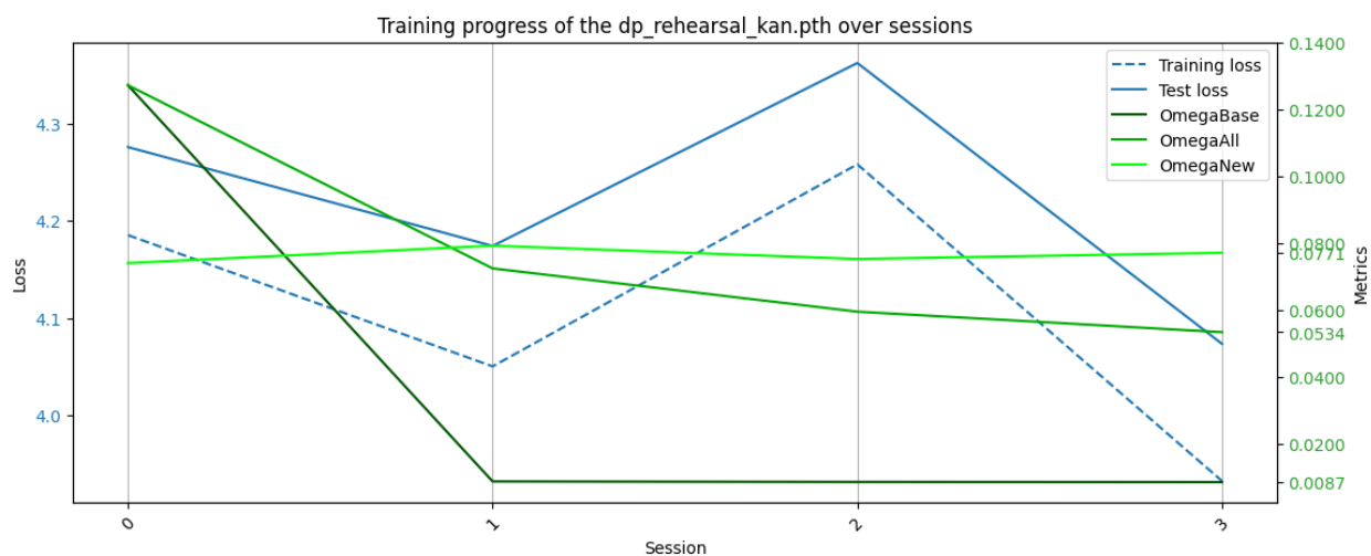
Приложение 9: График обучения KAN с адаптированным GeppNet в эксперименте с перестановкой признаков
