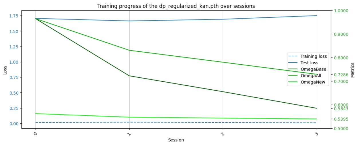
Приложение 8: График обучения KAN с адаптированным EWC в эксперименте с перестановкой признаков
