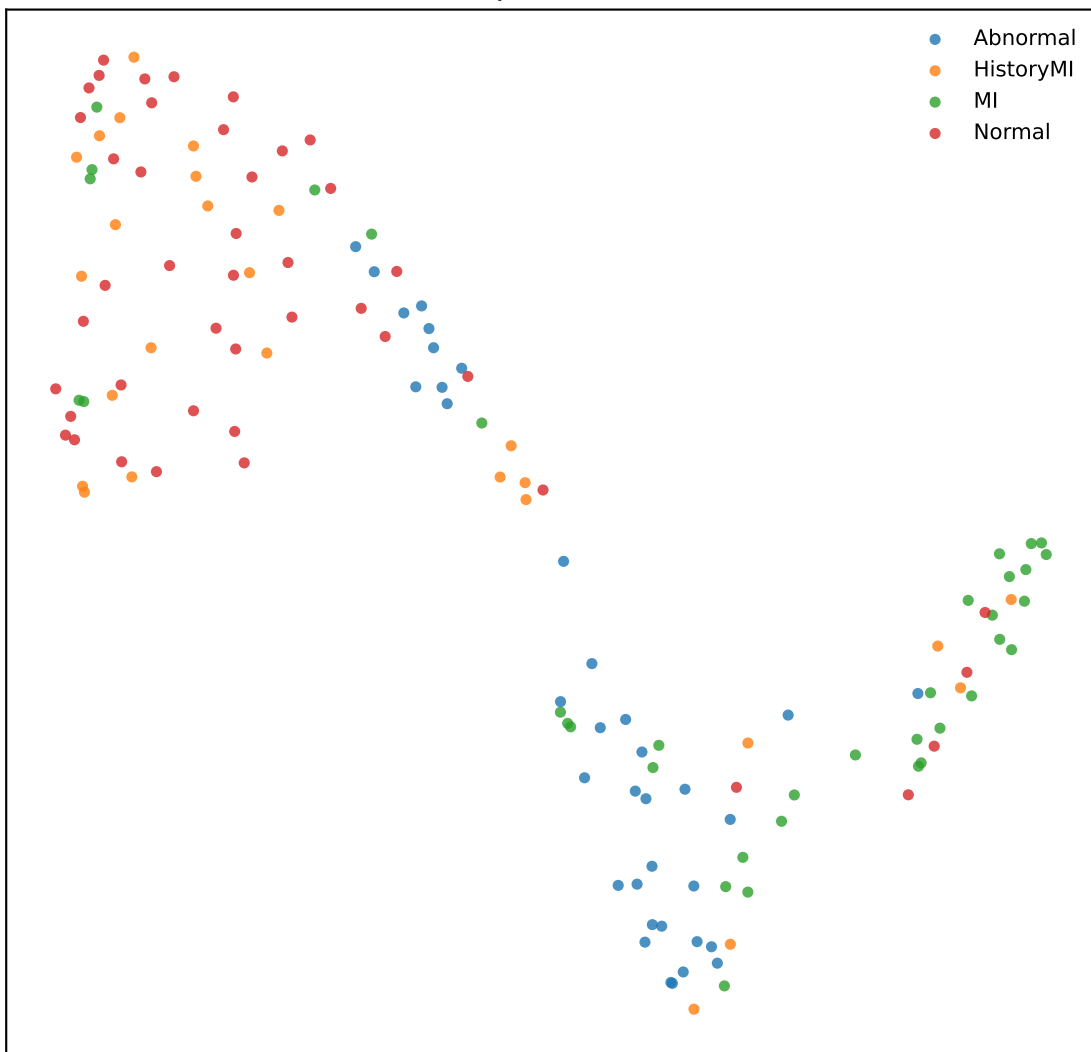
UMAP der Feature-Repräsentationen - resnet101
