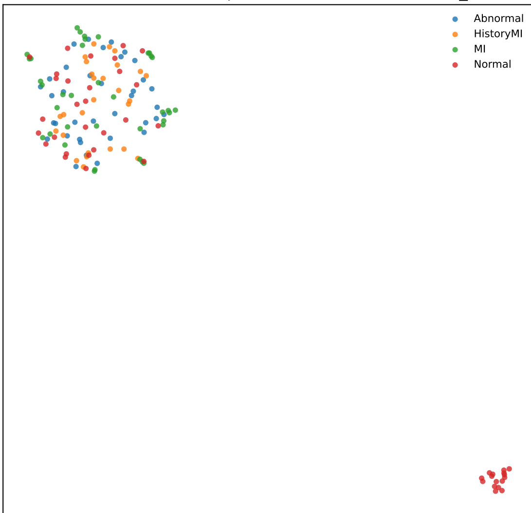
UMAP der Feature-Repräsentationen - mobilenet_v2
