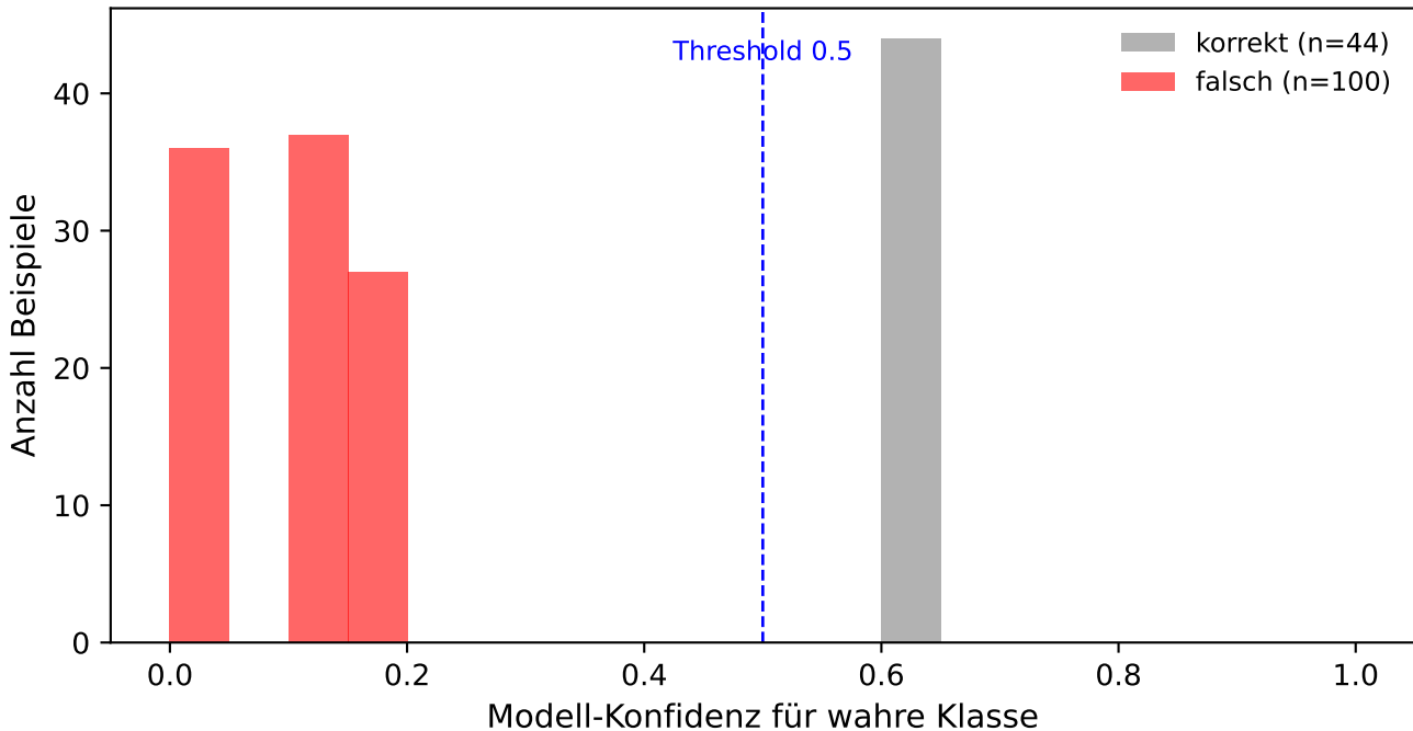
Verteilung der Konfidenz - mobilenet_v2 (Accuracy = 0.306)
