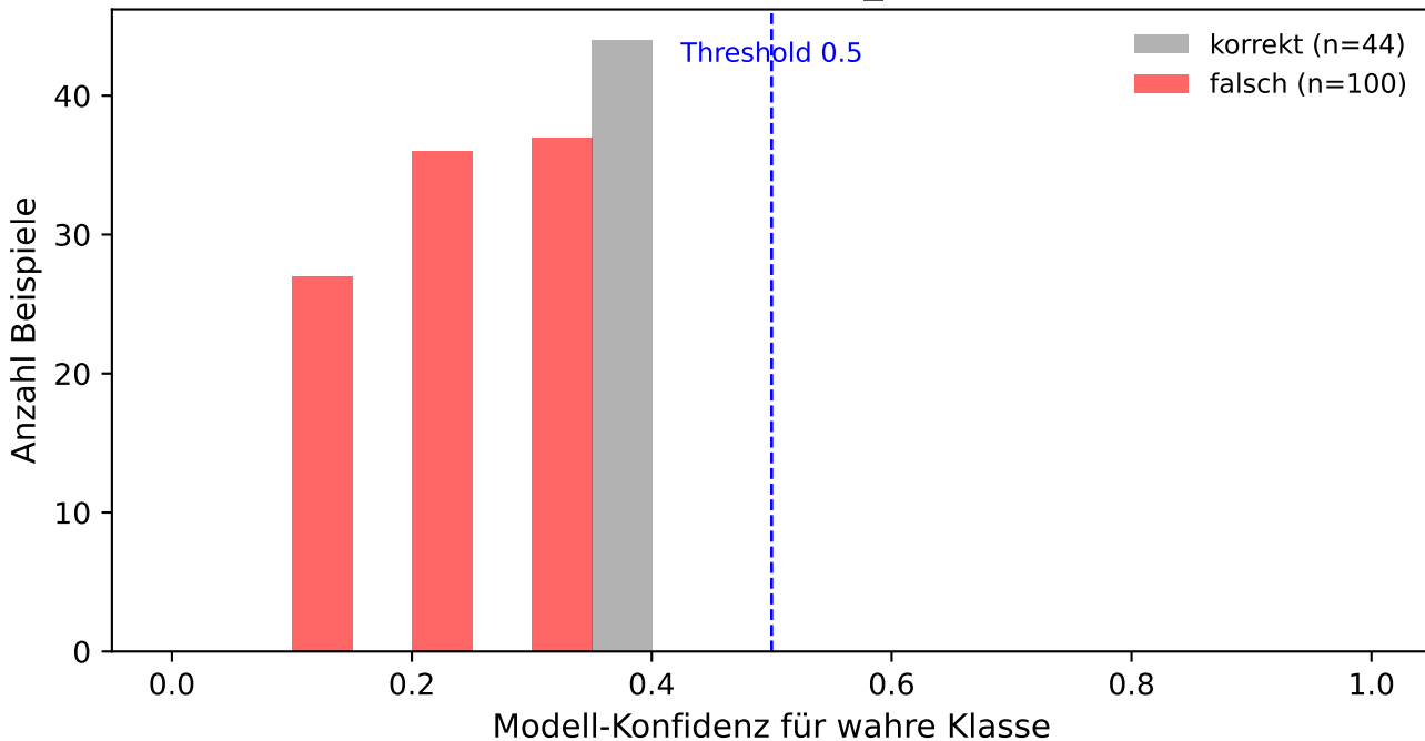
Verteilung der Konfidenz - vgg16_bn (Accuracy = 0.306)
