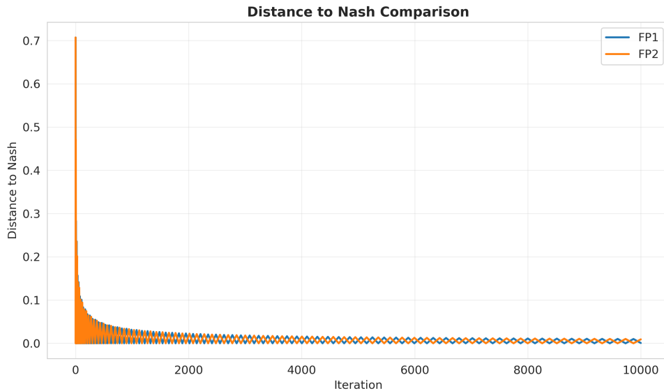
Σχήμα 2: Ευκλείδεια απόσταση της εμπειρικής στρατηγικής από το Nash (0.5, 0.5). Και οι δύο πράκτορες έχουν απόσταση κοντά στο 0.
