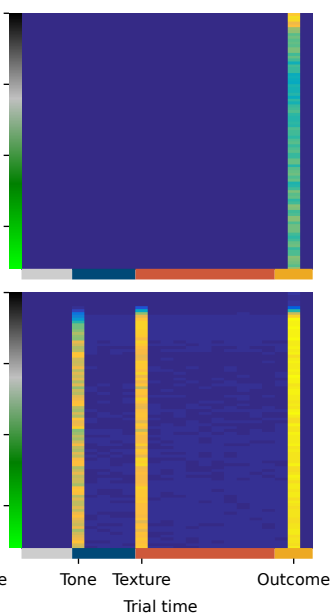
NoGo neuron
