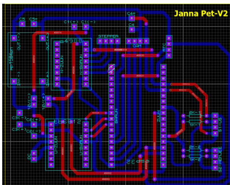
Зураг 2.9. Системийн РСВ дизайн
