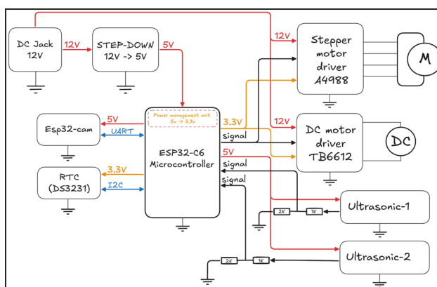
Зураг 2.1. Системийн ерөнхий архитектур
