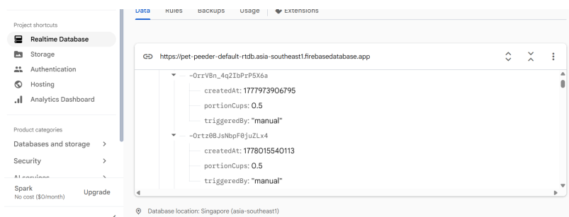
Зураг 2.6. Firebase Realtime Database-ийн бүтэц
