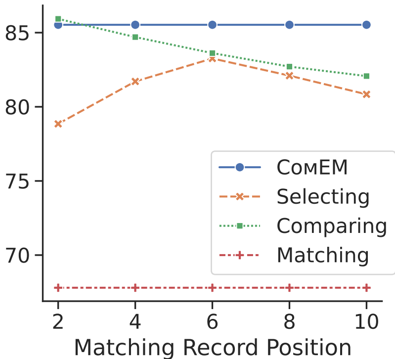
GPT-4o Mini
