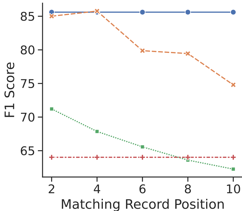
GPT-3.5 Turbo
