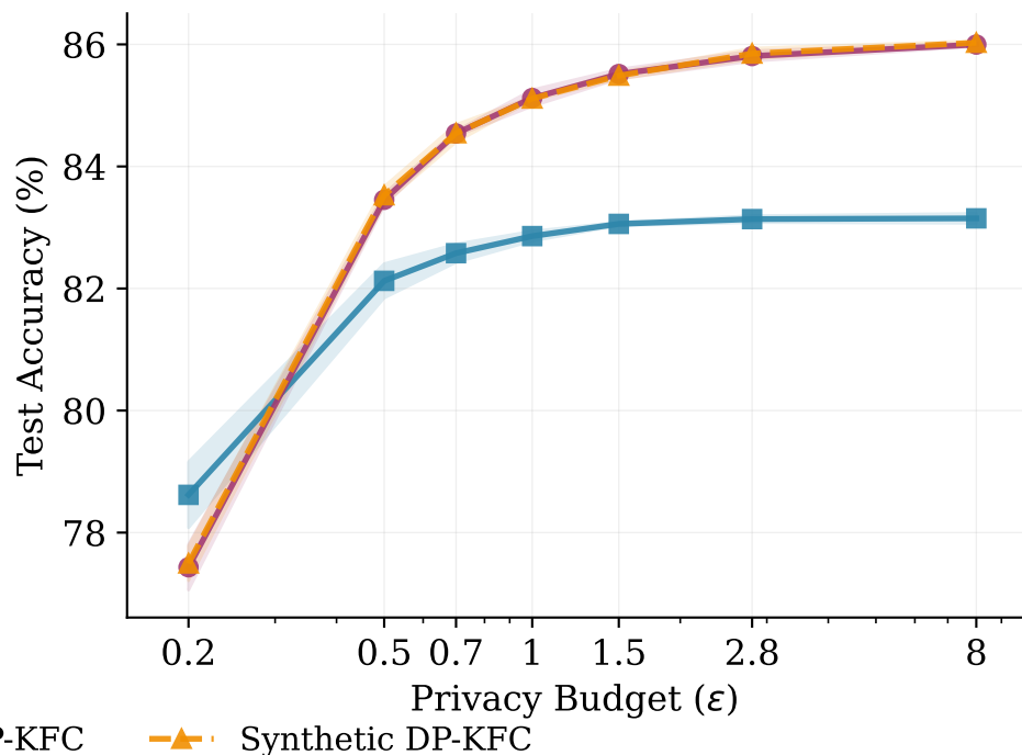
(b) IMDB
