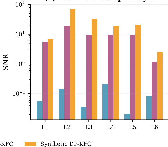
(b) CrossViT: SNR per Layer
