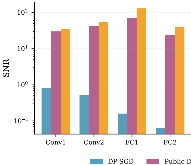
(a) CNN: SNR per Layer
