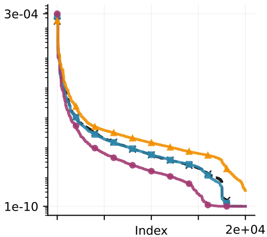
CNN: conv
