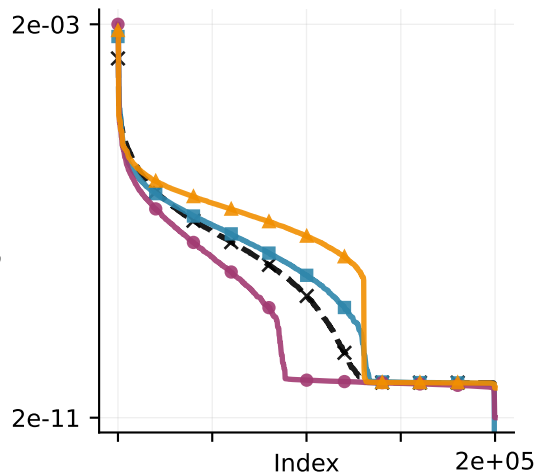
MLP: fc
