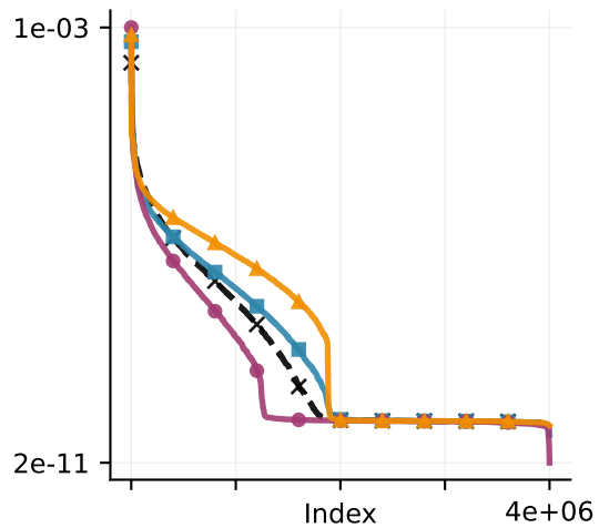
Attn: qkv
