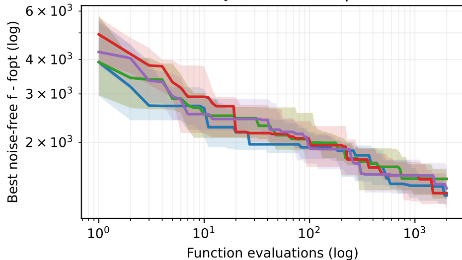
bbob-noisy f14 (id=114) | D=40
