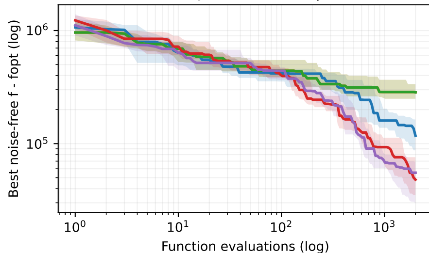
bbob-noisy f10 (id=110) | D=40
