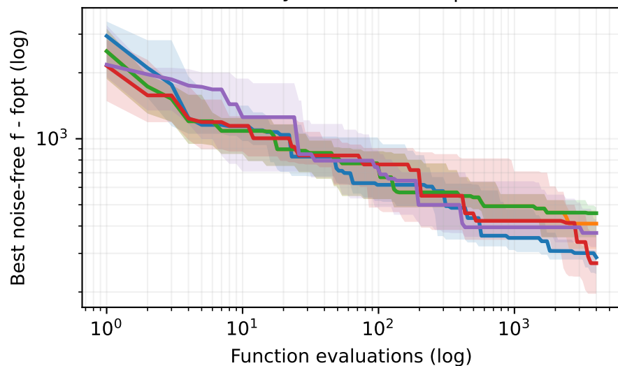
bbob-noisy f14 (id=114) | D=20
