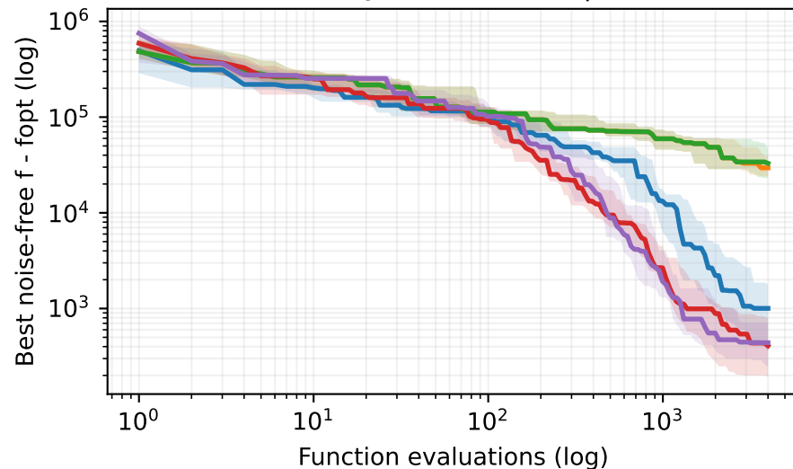
bbob-noisy f10 (id=110) | D=20
