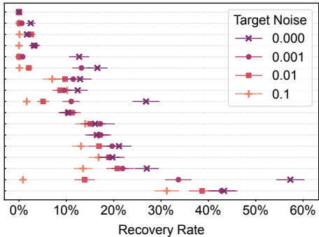
Feynman Dataset
