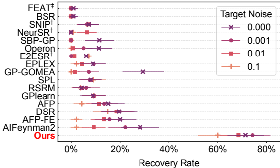
Strogatz Dataset
