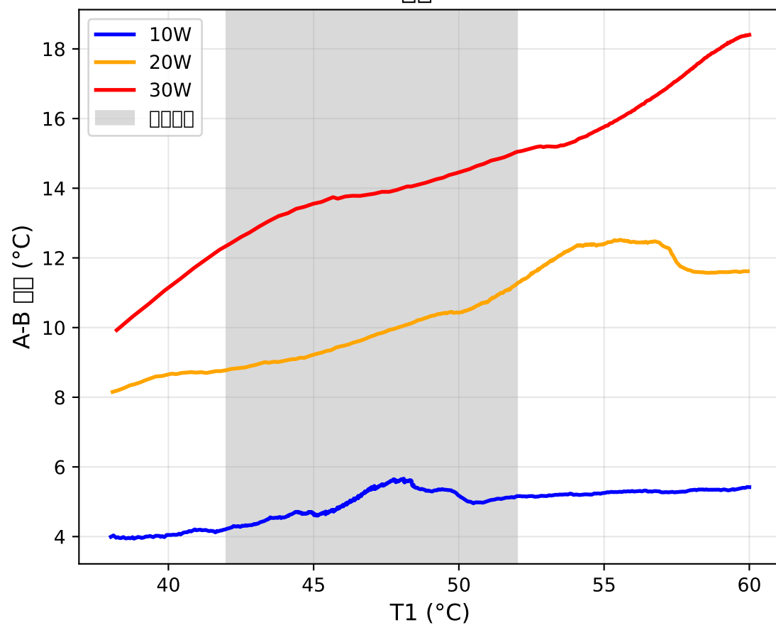
\Delta T -T1
