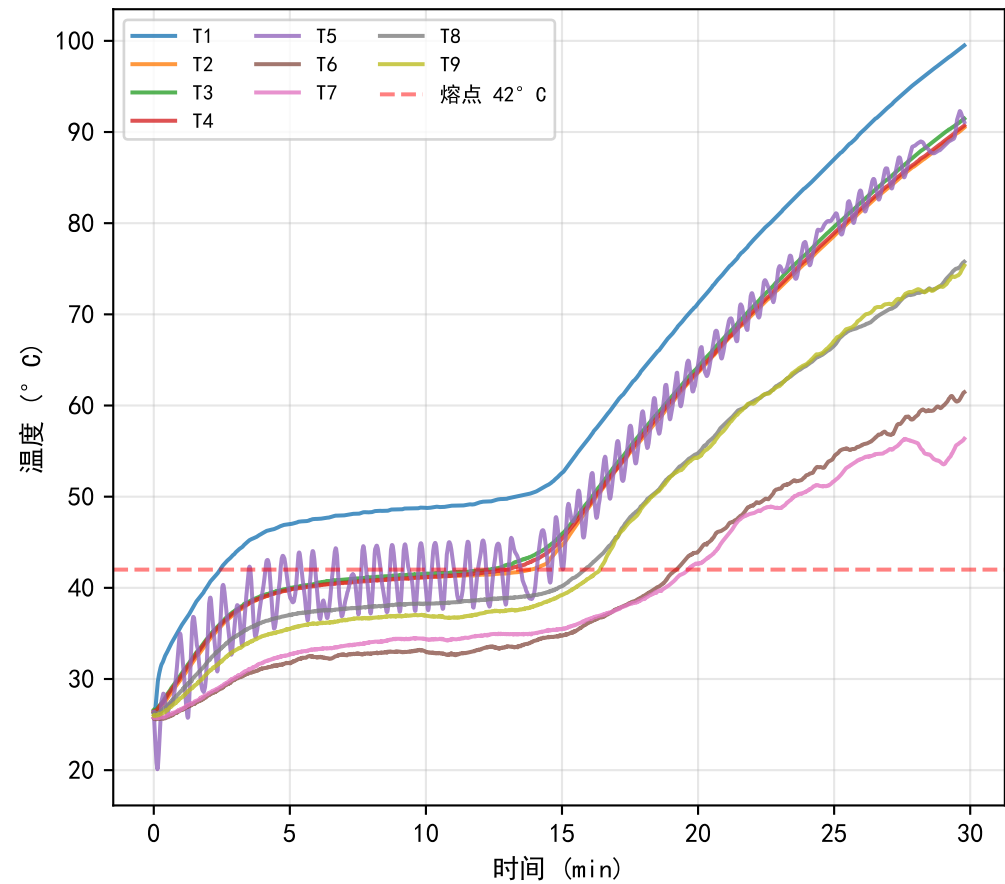
IWP 10W 所有传感器温度曲线
