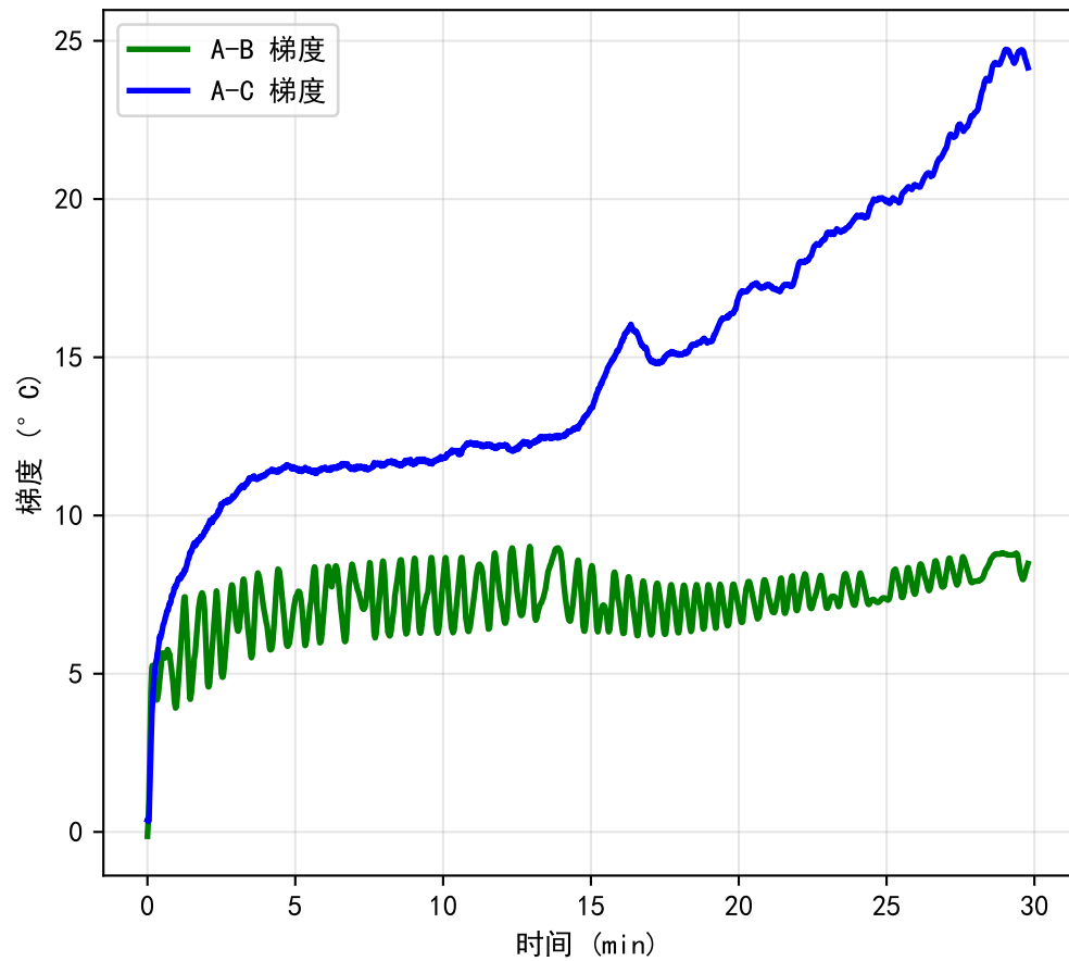
IWP 10W 温度梯度随时间变化
