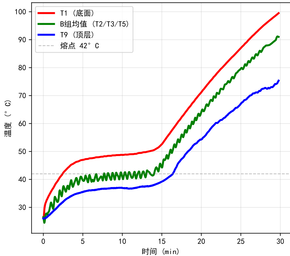
IWP 10W 关键位置温度对比
