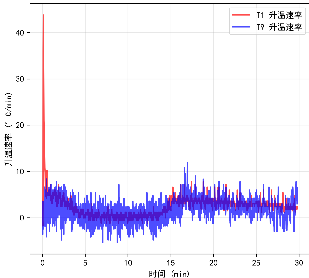
IWP 10W 升温速率
