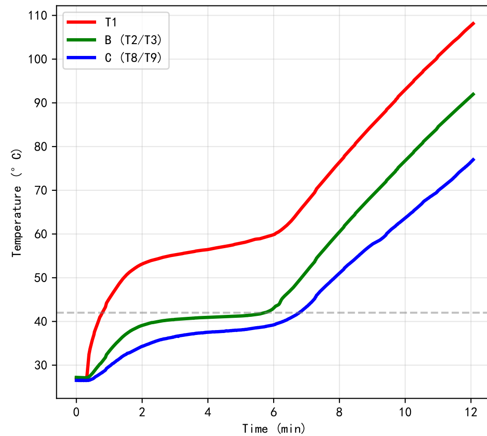
IWP 20W A-C Gradient vs T1
