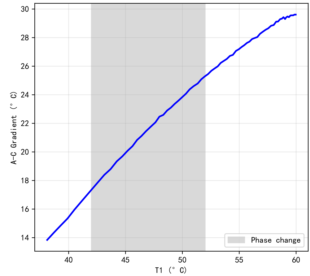
IWP 30W A-C Gradient vs T1
