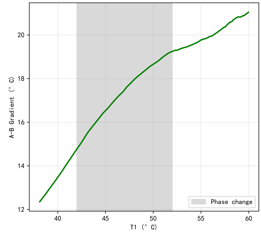
IWP 30W A-B Gradient vs T1
