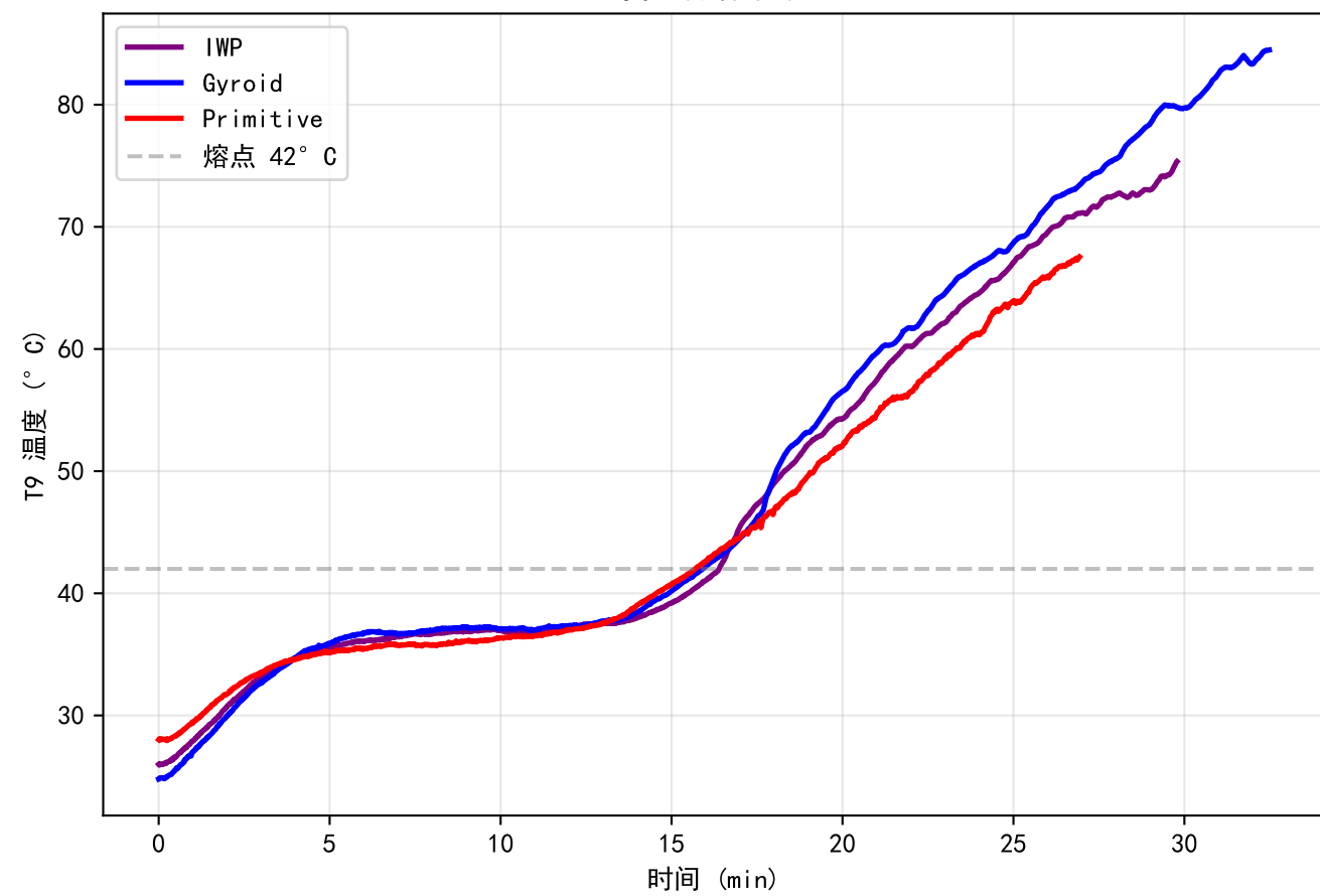
T9 温度-时间曲线 (10W)
