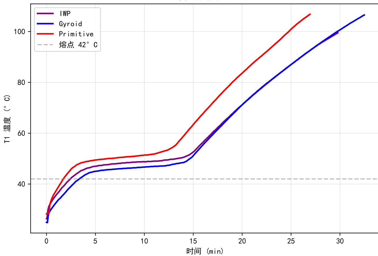
T1 温度-时间曲线 (10W)
