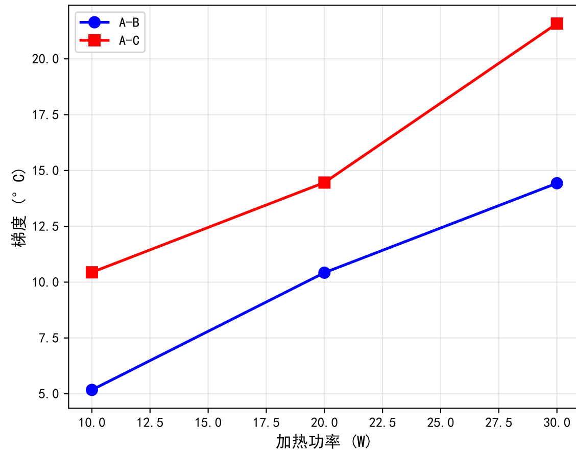
T1=50 ^{\circ}\text{C} 时梯度 vs 功率
