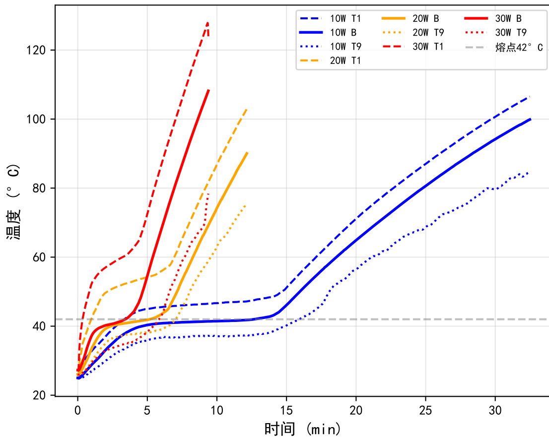
温度-时间曲线
