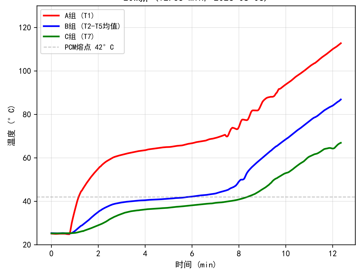
20W新 温度梯度
