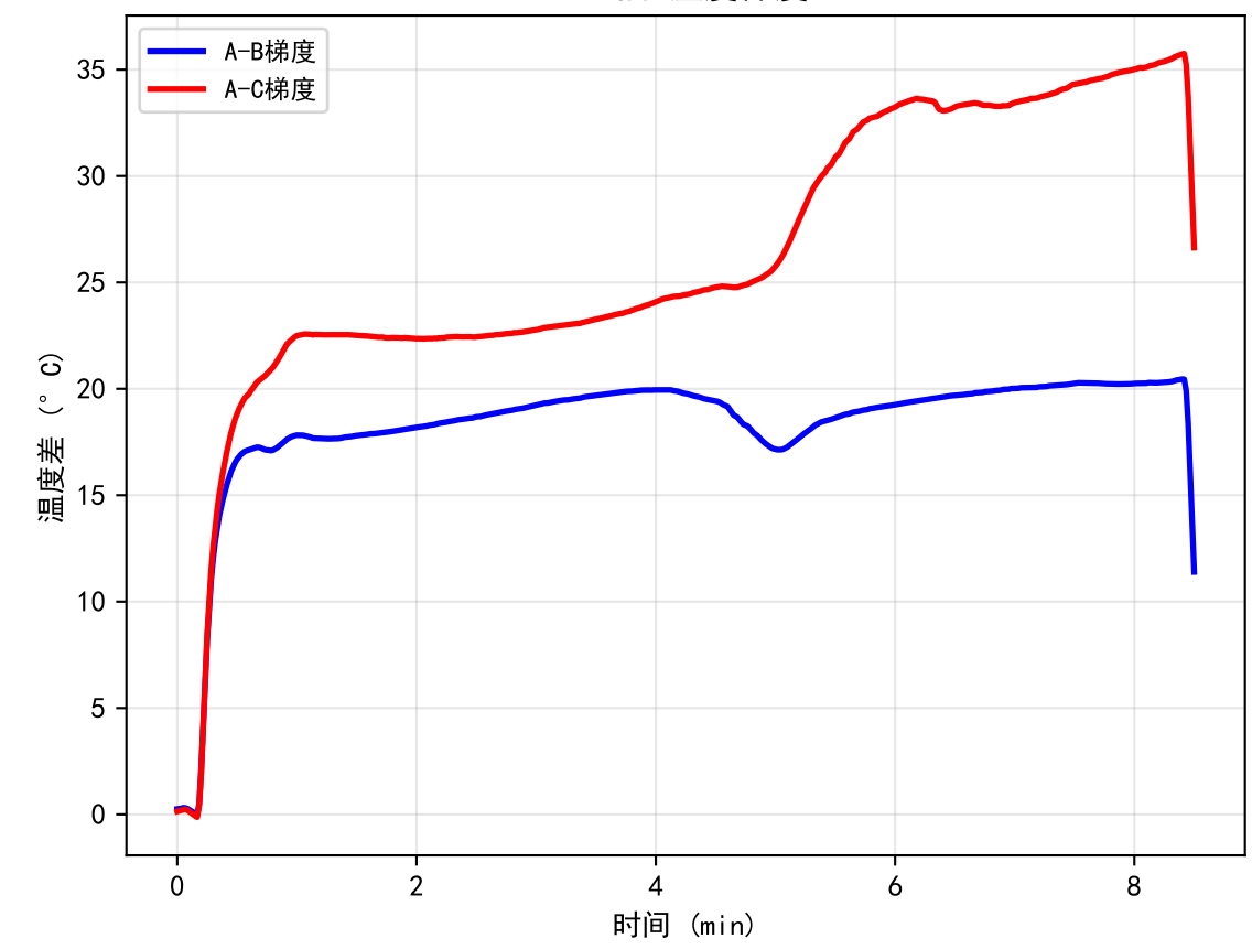
20W旧 温度梯度
