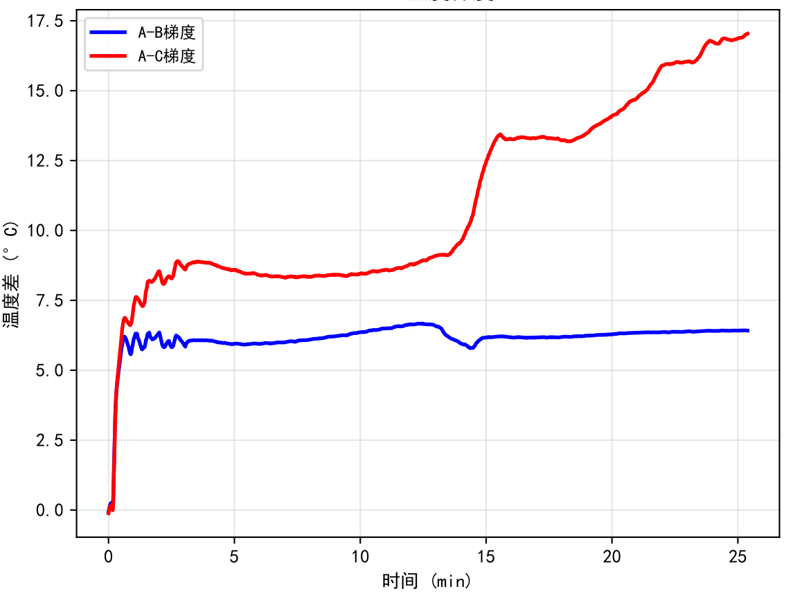
10W 温度梯度
