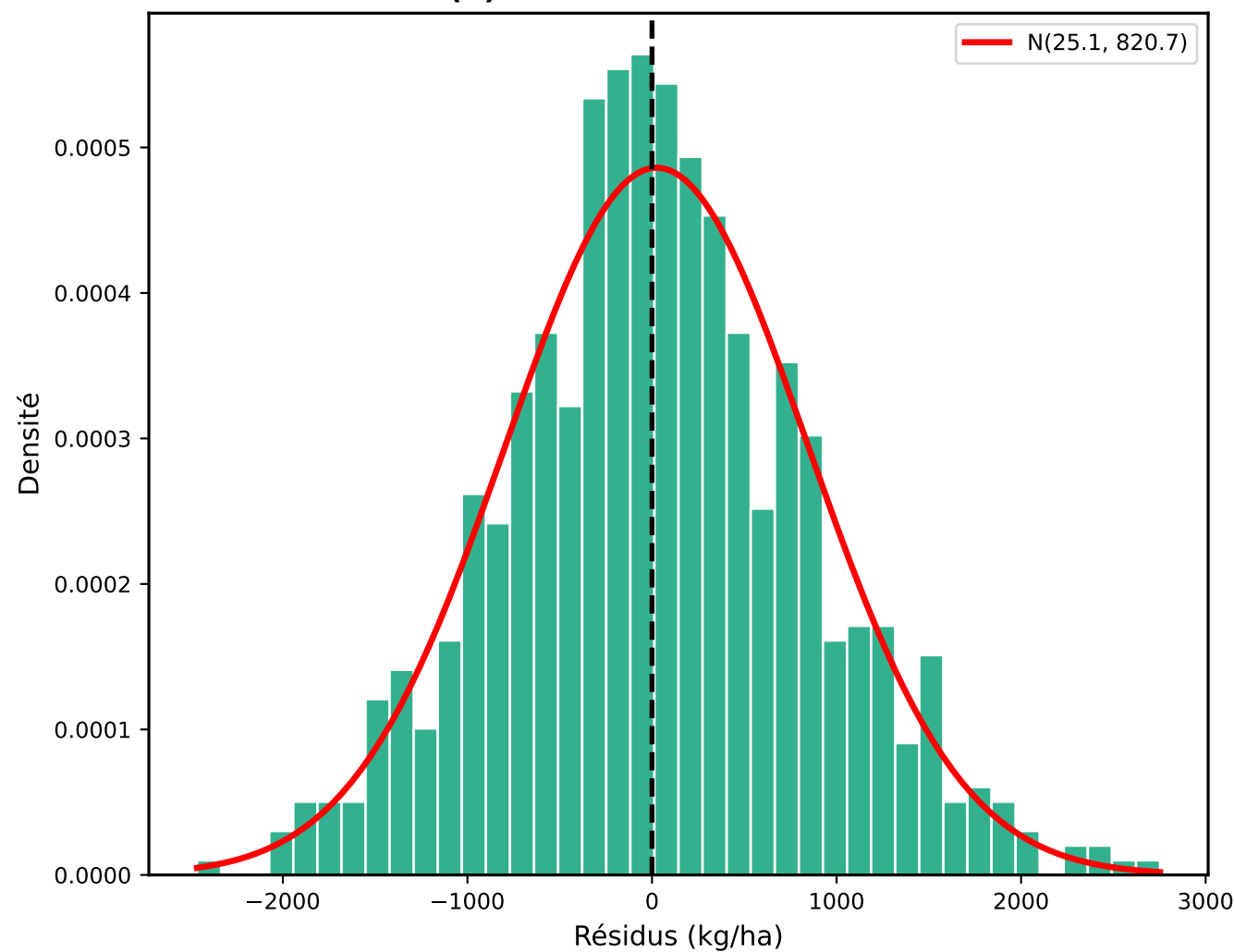
(C) Distribution des résidus
