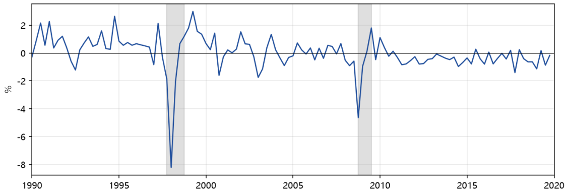
그림 4.5: 관측변수: 한국 1인당 실질 GDP 증가율(평균 제거, 1990Q1~2019Q4). 음영은 외환위기와 글로벌 금융위기.
