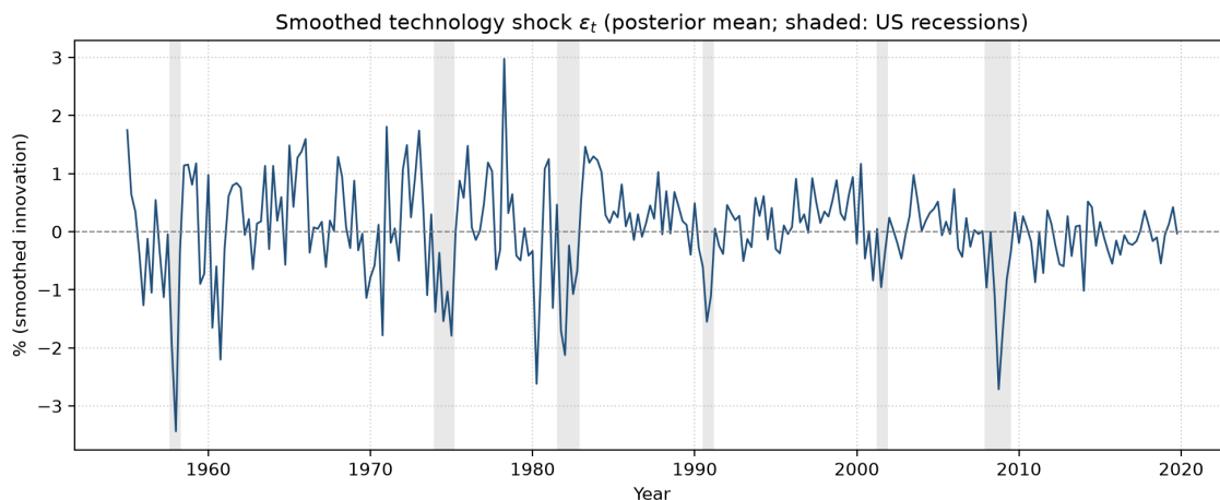
그림 4.4: 평활화된 기술충격 \hat{\varepsilon}_t (사후 평균). 음영은 미국의 경기침체기.
