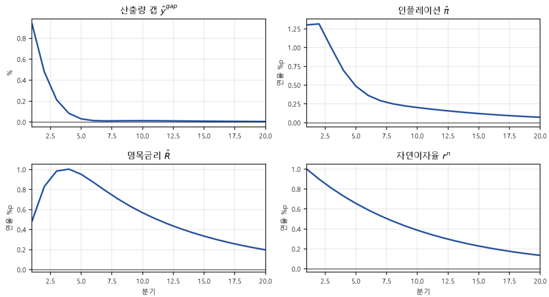
그림 6.1: 수요 충격(자연이자율 연율 +1%p, \rho_n = 0.9 )에 대한 충격반응. 산출량 갭은 %, 금리·인플레이션은 연율 %p 편차이다.
