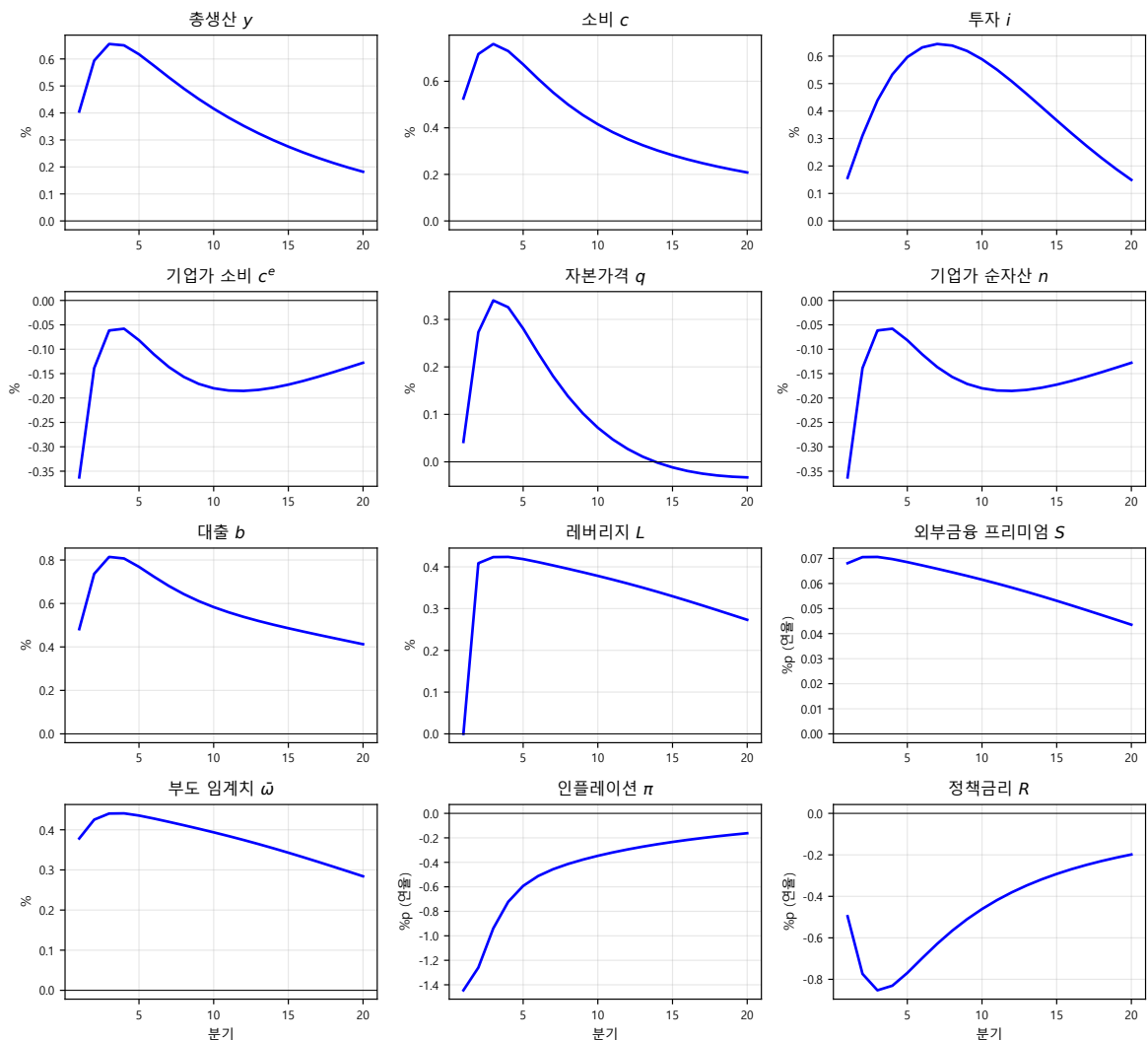
그림 14.3: 기술 충격(+1%)에 대한 충격반응.
