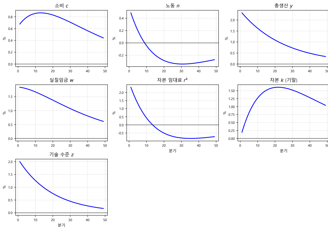
그림 A.1: 기술충격(+2%)에 대한 충격반응 (Python 섭동법 풀이). 세로축은 정상상태 대비 % 편차이다.
