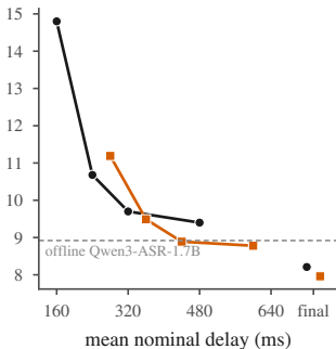
(b) Kspon clean (Ko), CER %
