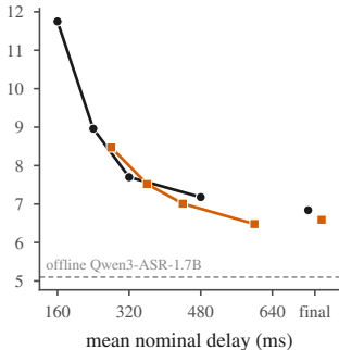
(a) VoxPopuli-AA (En), WER %
