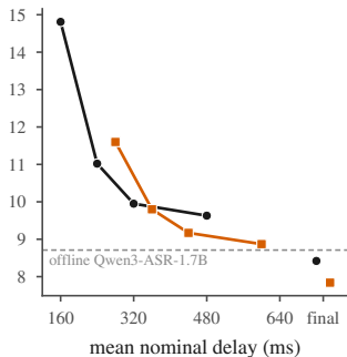
(c) Kspon other (Ko), CER %
