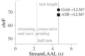
(a) En→De
