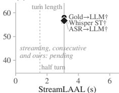
(b) De→En
