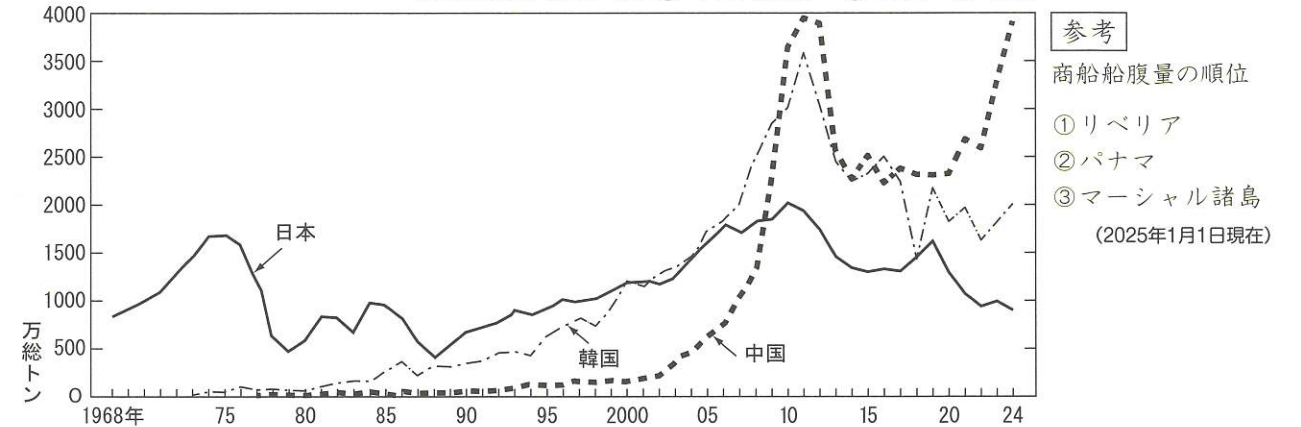
図 12 世界の造船竣工量
