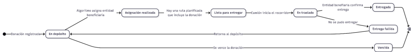
Figura 2 - Diagrama de Estados de una donación.
