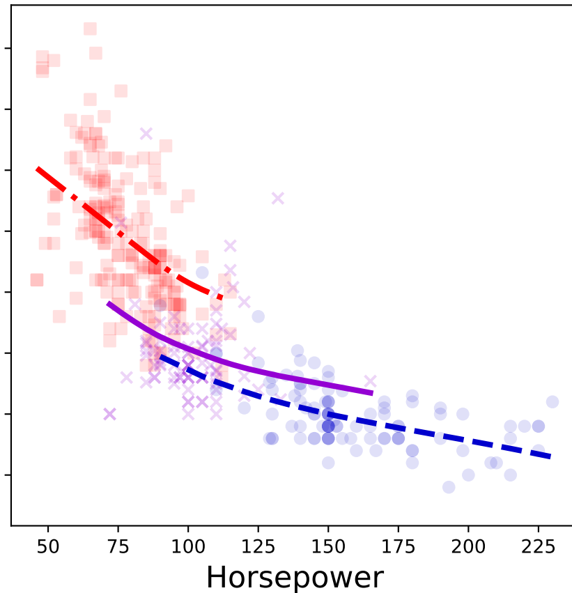
LiD-GLM
