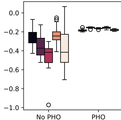
origin_3
