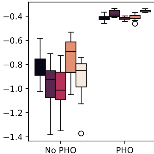
origin_2
