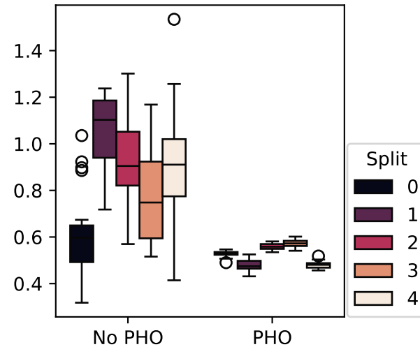
origin_3
