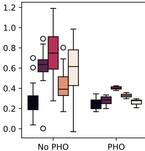
origin_2
