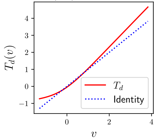
(a.1) T_d : \mathbb{R} \rightarrow \mathbb{R}
