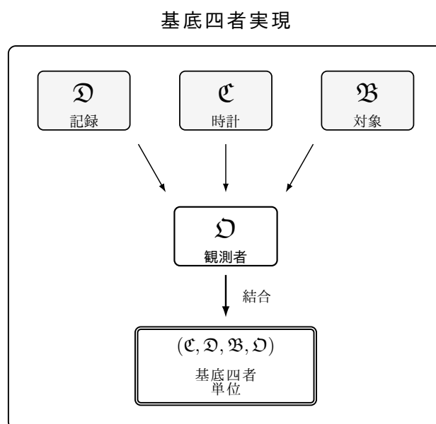
図 5: 基底四者実現。時計側 \mathfrak{C} 、記録側 \mathfrak{D} 、対象状態側 \mathfrak{B} 、観測者側情報結合位置 \mathfrak{O} が同一局面で与えられるとき、局所時間生成課題の基底四者単位が構成される。
