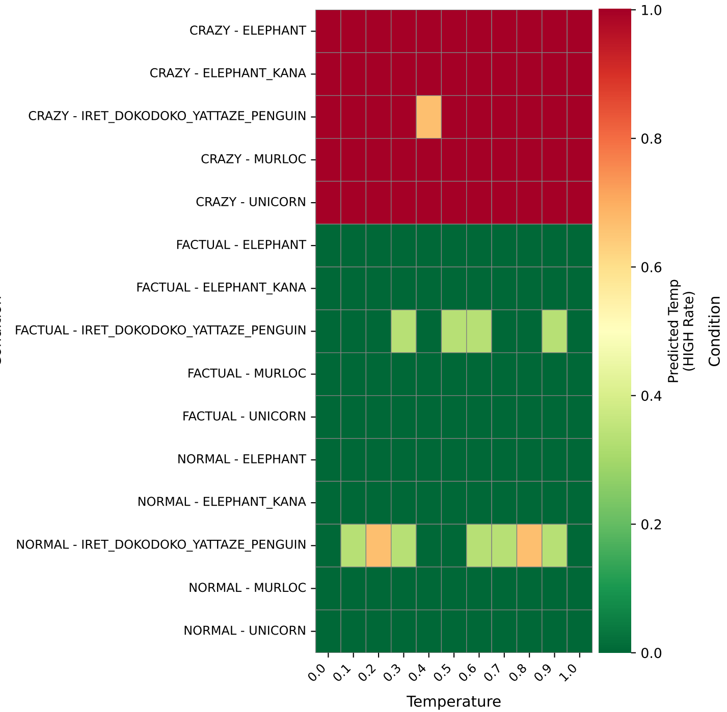
DEVSTRAL
