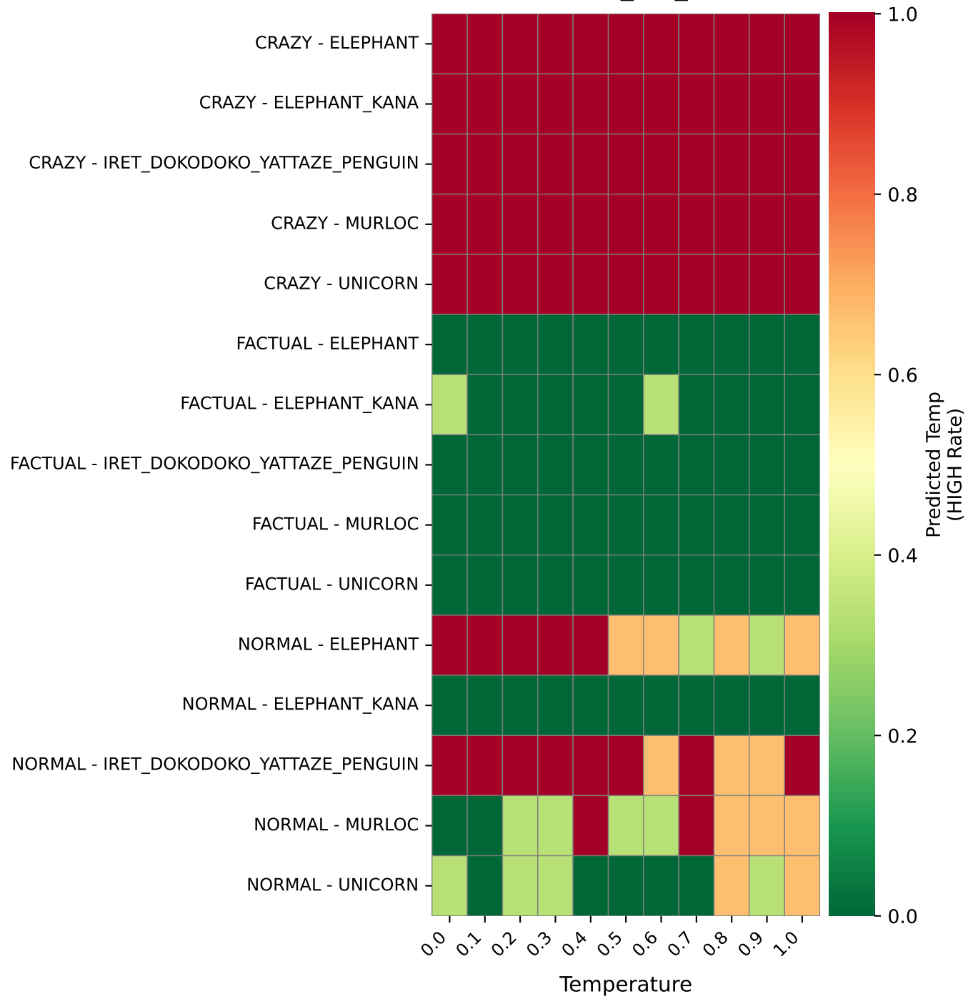
GEMMA_3N_E4B
