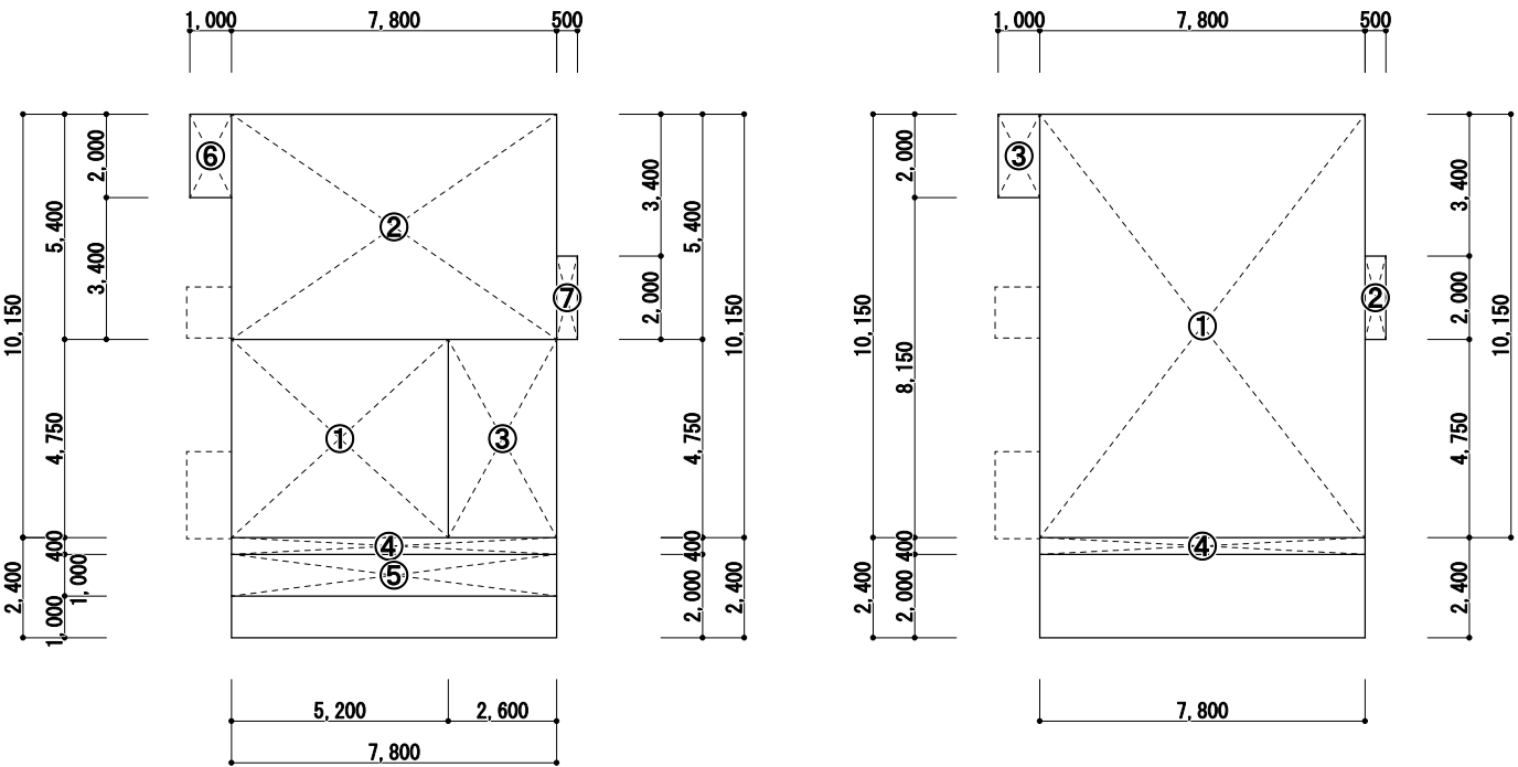
1階平面図 S=1/200
