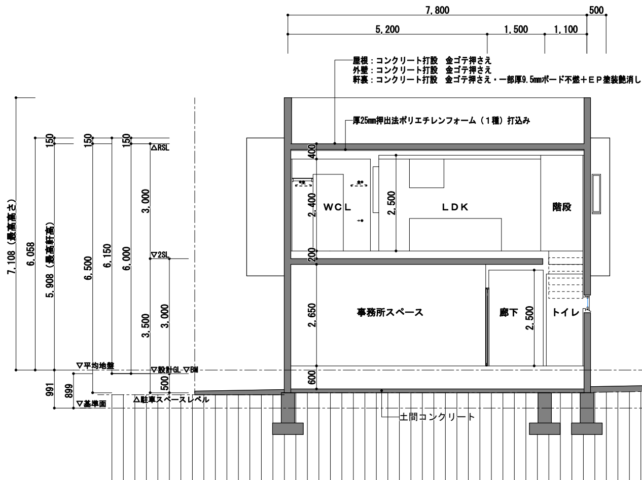
A-A断面図 S=1/100
