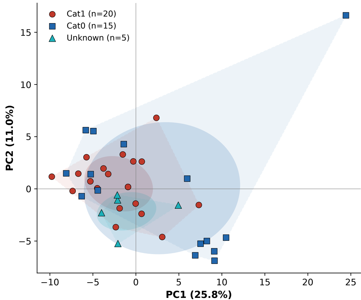
b 168 extended RDKit descriptors
