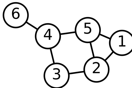
図1 単純グラフ
