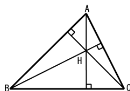
図 5 三角形の垂心
