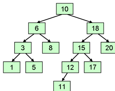
図2 にぶんたんさくぎ 二分探索木
