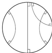
図8 ポアンカレディスクモデル
