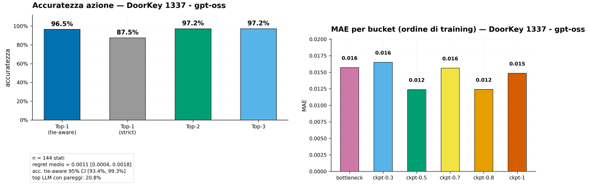
Figura 5: Il pannello sinistro mostra la selezione Top-k aggregata sui 144 stati validi dello scenario di base: Top-1 tie-aware 96.5%, Top-1 strict 87.5%, Top-2 97.2% e Top-3 97.2%. Il pannello destro è un MAE per bucket, non un grafico Top-k: le barre sono in ordine di training, cioè da meno a più step di addestramento, con bottleneck 0.0157, ckpt-0.3 0.0165, ckpt-0.5 0.0124, ckpt-0.7 0.0156, ckpt-0.8 0.0124 e ckpt-1 0.0148. I due pannelli descrivono rispettivamente accuratezza dell'azione ed errore numerico.
