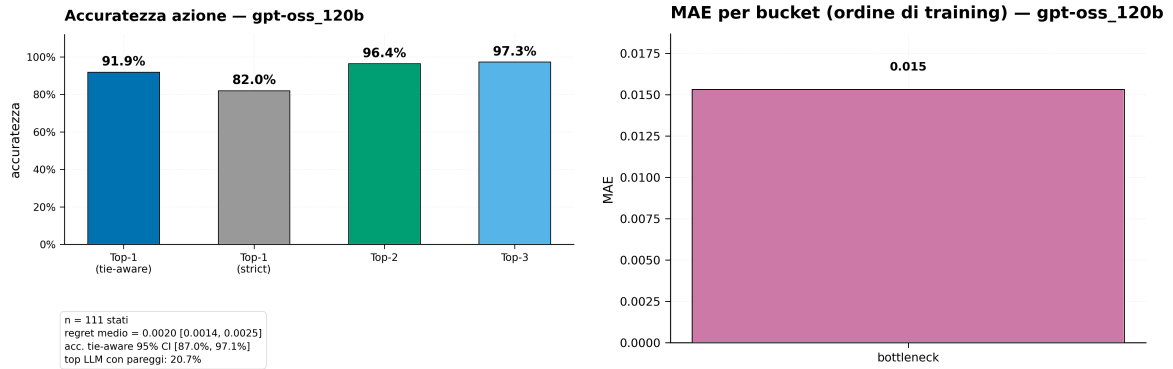
Figura 6: Il pannello sinistro mostra la selezione Top-k aggregata sui 111 stati validi dei cinque layout: Top-1 tie-aware 91.9%, Top-1 strict 82.0%, Top-2 96.4% e Top-3 97.3%. Il pannello destro è il MAE per bucket e mostra soltanto bottleneck , con valore 0.015; non presenta una barra per ciascuna tipologia di stato. I valori Top-k e il MAE per bucket non vanno confusi.
