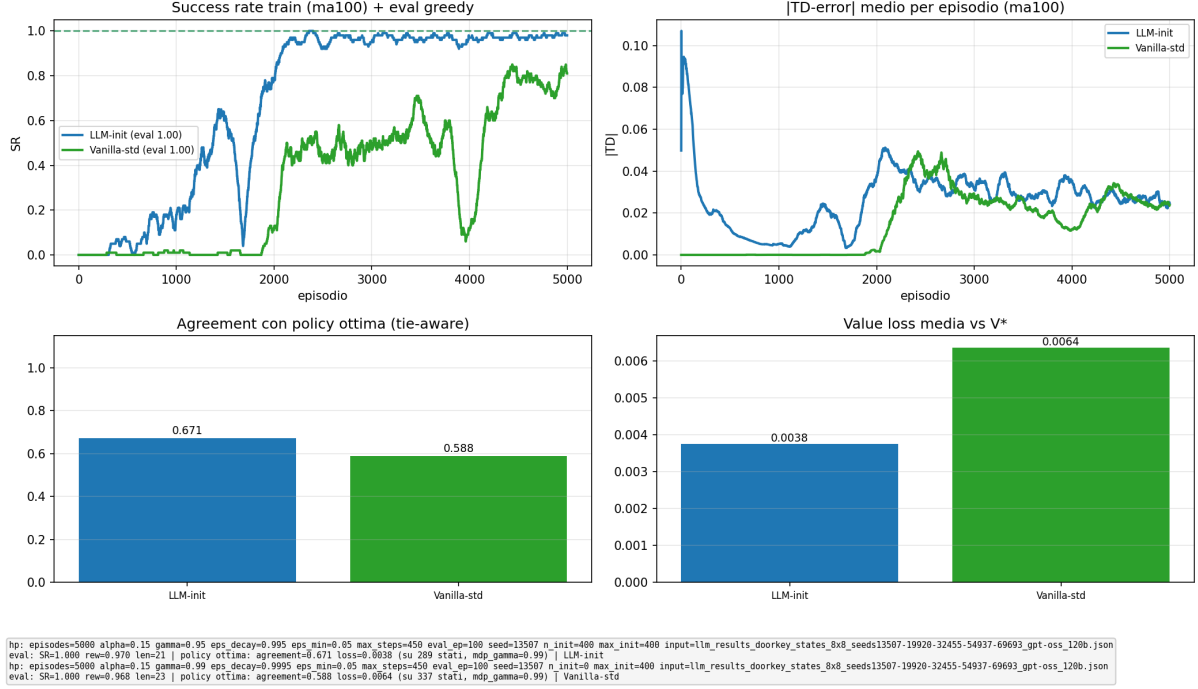
Figura 11: Il confronto tra LLM-init e Vanilla-std mostra gli stessi quattro pannelli del run da 5000 episodi, con LLM-init configurato con \alpha = 0.15 e il controllo standard con \alpha = 0.15 e \gamma = 0.99 . Anche in questo caso la valutazione riportata è sul seed 13507, presente nell’addestramento, e non sul seed non visto 69694. I valori finali riportati per LLM-init sono SR=1.000, len=21, agreement=0.671 e loss=0.0038; per Vanilla-std sono SR=0.000, len=450, agreement=0.587 e loss=0.0067. Il grafico non mostra quindi un test di generalizzazione su una mappa non vista.
