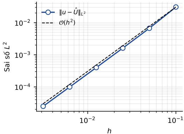
Chuẩn L^2 — bậc 2
