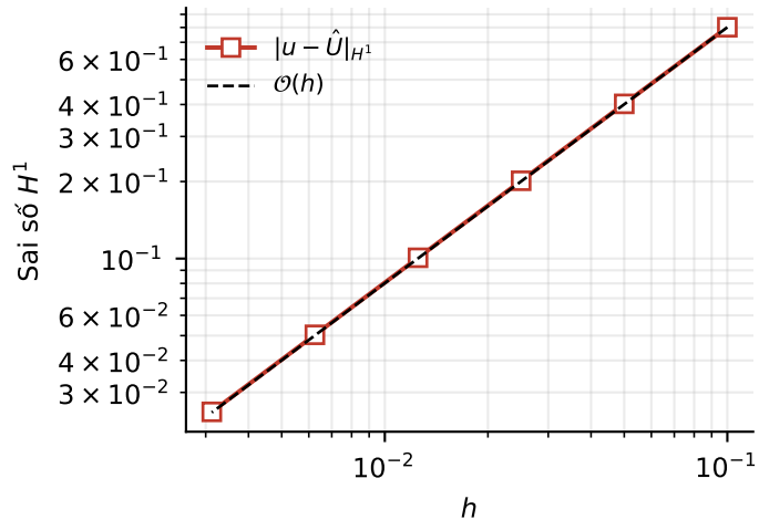
Nửa chuẩn H^1 — bậc 1
