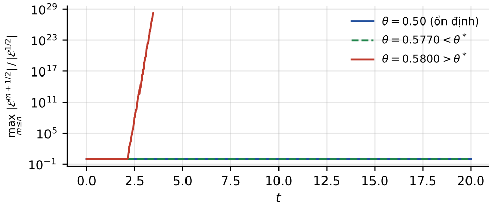
Bao trên của năng lượng rời rạc ( N = 80 )
