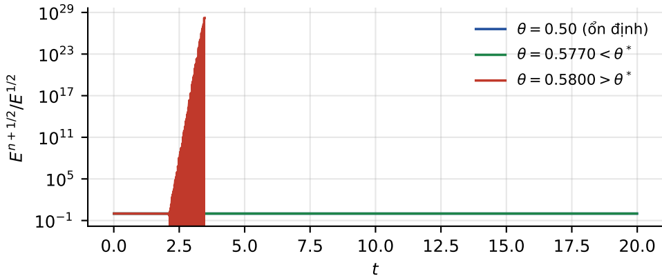
Năng lượng rời rạc theo thời gian ( N = 80 )
