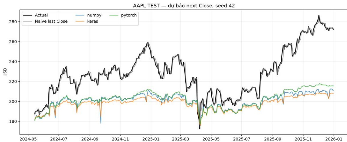
Hình 4.5. AAPL TEST actual-vs-predicted của seed 42; naive bám sát actual hơn ba RNN
