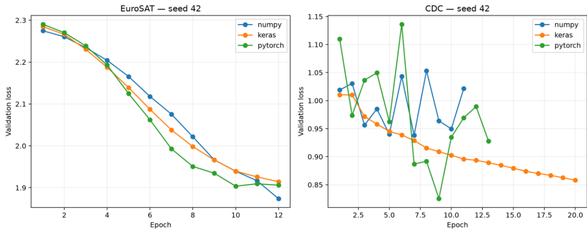
Hình 3.4. Validation loss của matched CNN ở seed 42
