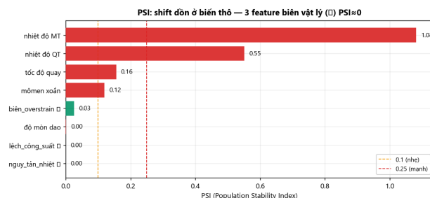
Hình 6. Chỉ số PSI: dịch chuyển tập trung ở biến thô; ba đặc trưng biến có PSI xấp xỉ 0.
