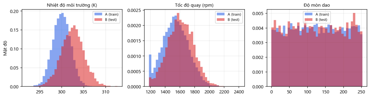
Hình 1. Phân phối chồng lấn giữa Dây chuyền A và B: nhiệt độ và tốc độ dịch chuyển rõ rệt, trong khi độ mòn dao ổn định.
