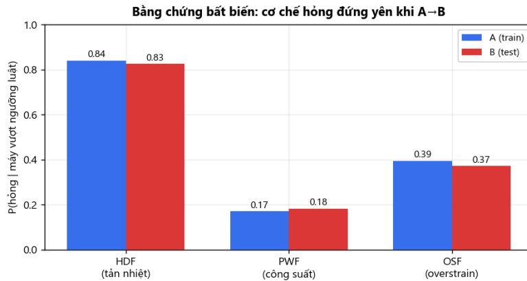
Hình 8. Xác suất hỏng có điều kiện P(\text{hỏng} \mid \text{vượt ngưỡng}) gần như không đổi khi chuyển từ A sang B, xác nhận cơ chế sinh lỗi bất biến.
