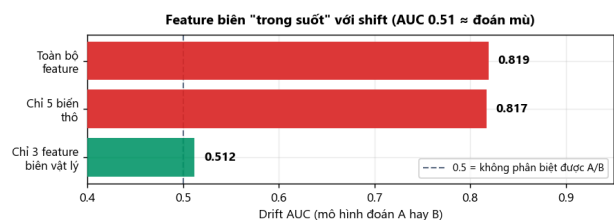
Hình 7. Drift-AUC: đặc trưng biến không phân biệt được A và B (0,51 ≈ dự đoán ngẫu nhiên).
