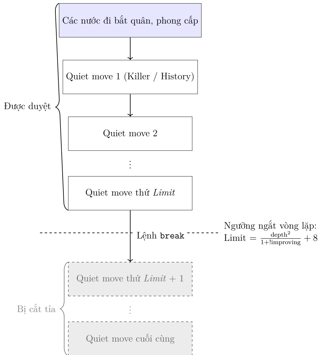
Hình 4.16: Minh họa cơ chế Cắt tĩa nước đi muộn (LMP).
