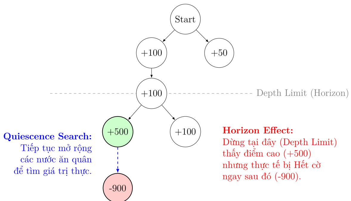
Hình 4.9: Minh họa Horizon Effect và Tìm kiếm tĩnh
