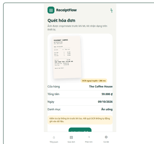
Hình 2. Kết quả OCR cần được kiểm tra trước khi lưu.
