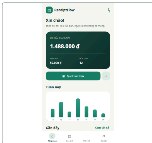
Hình 1. Dashboard tháng, tuần và giao dịch gần đây.
