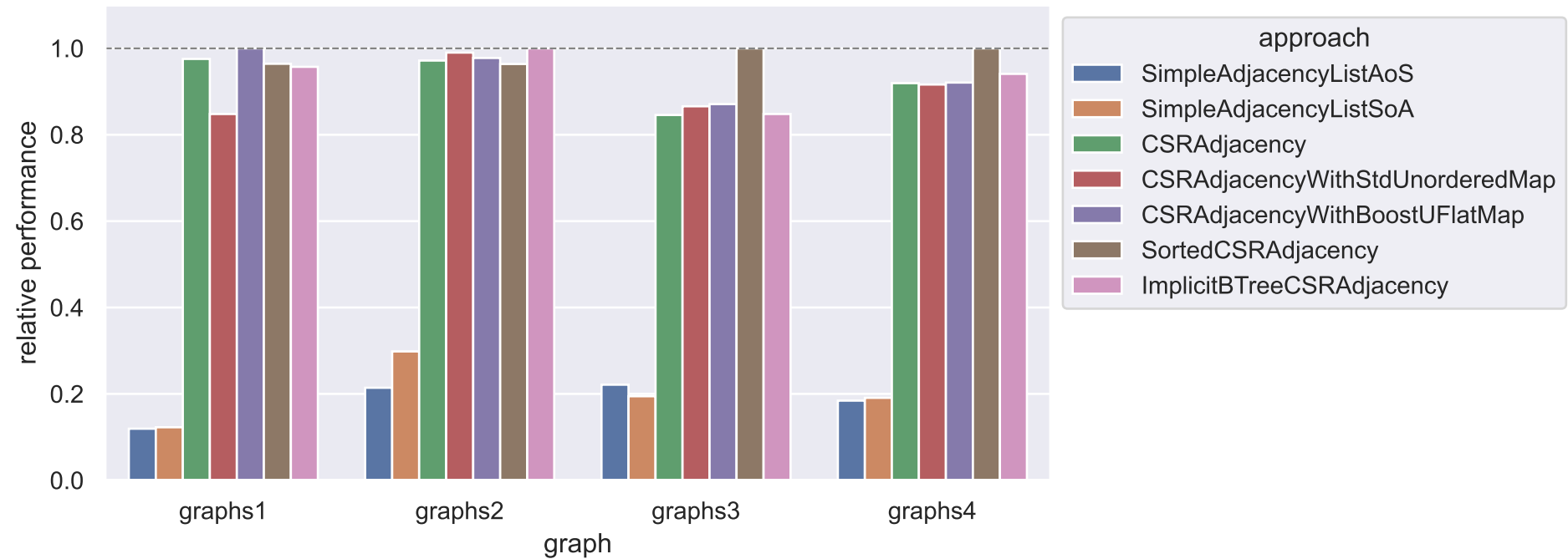
iterate_all_pairs
