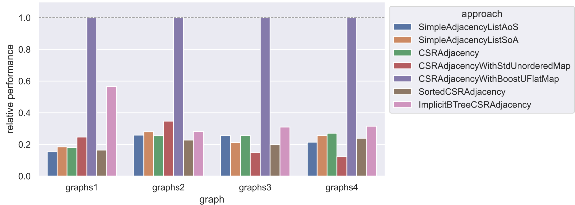
query_random_pairs
