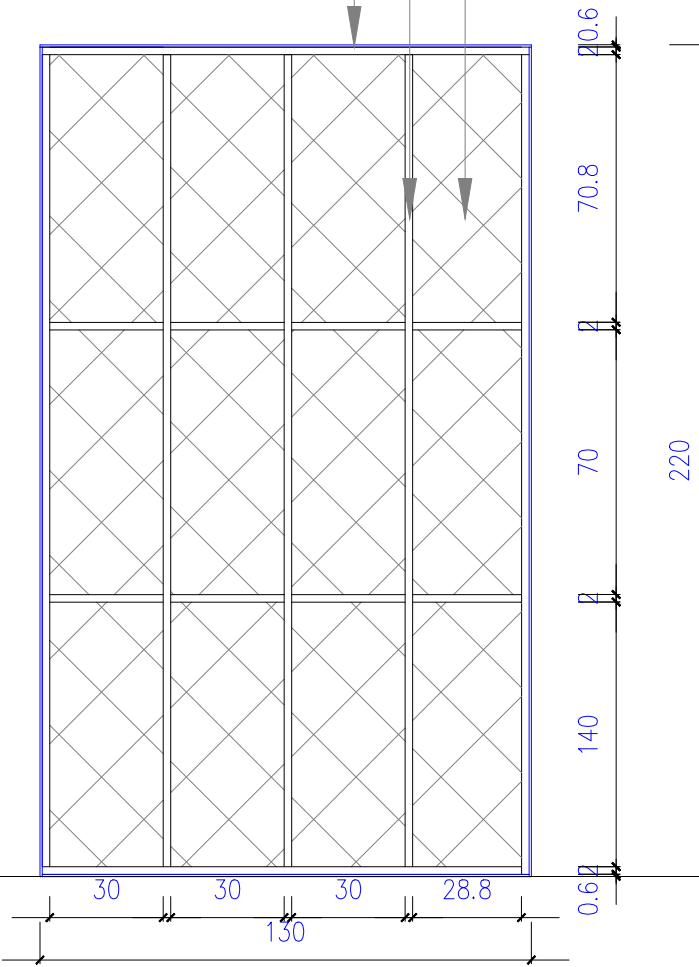
D8鉛門剖面圖▶
