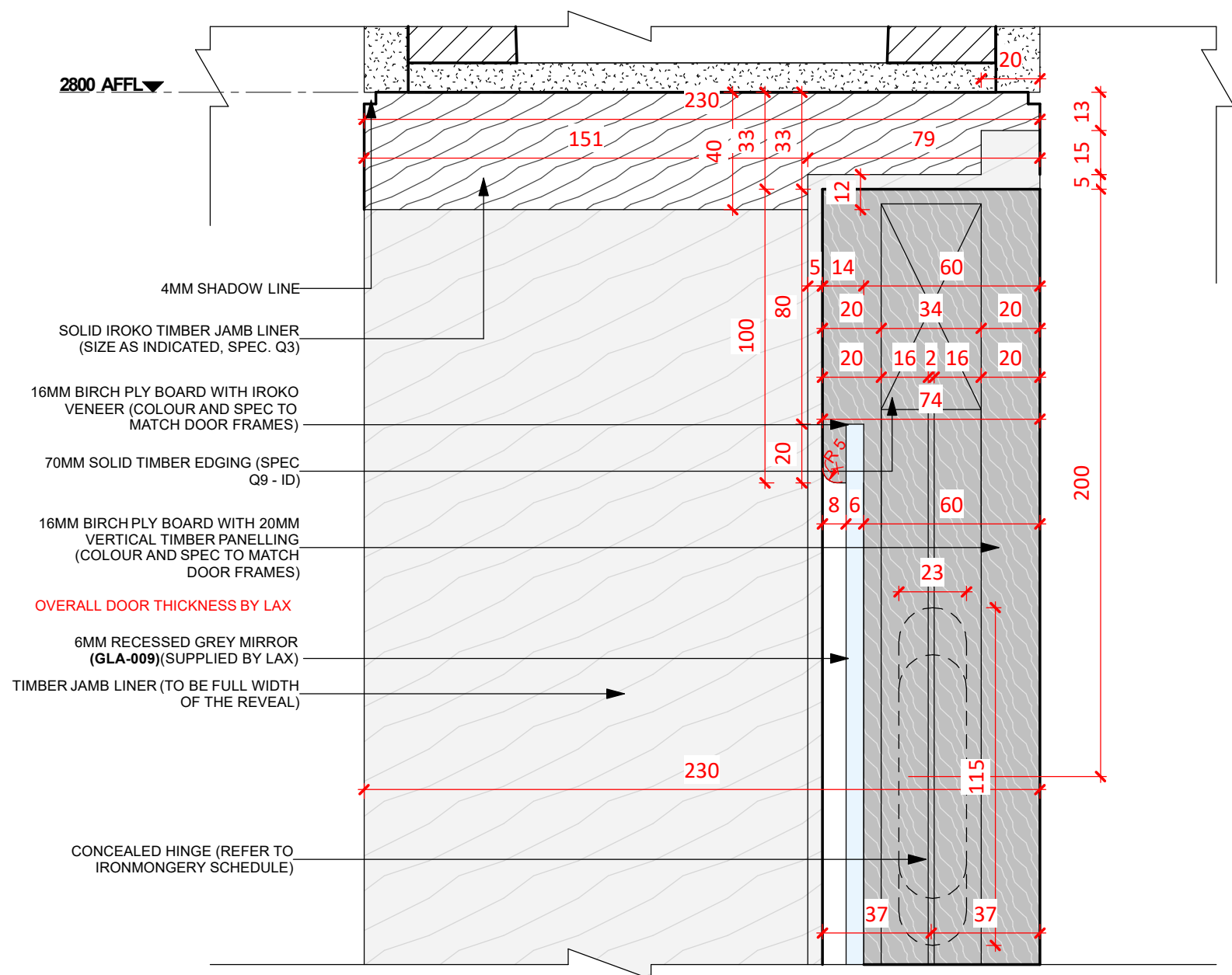
Hinge Door Detail Section - Top of Door | 1:2
