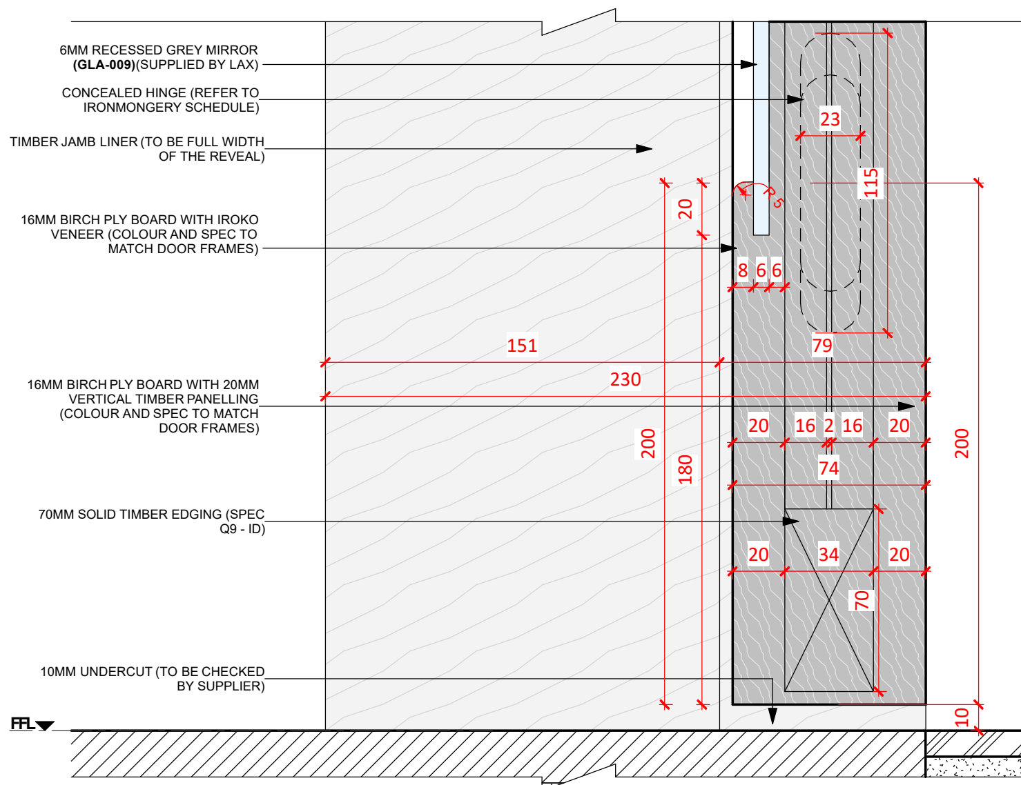
Hinge Door Detail Section - Top of Door | 1:2
